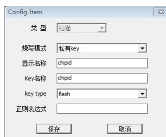
图 7-5: DragonSn 烧录私有 key 配置
