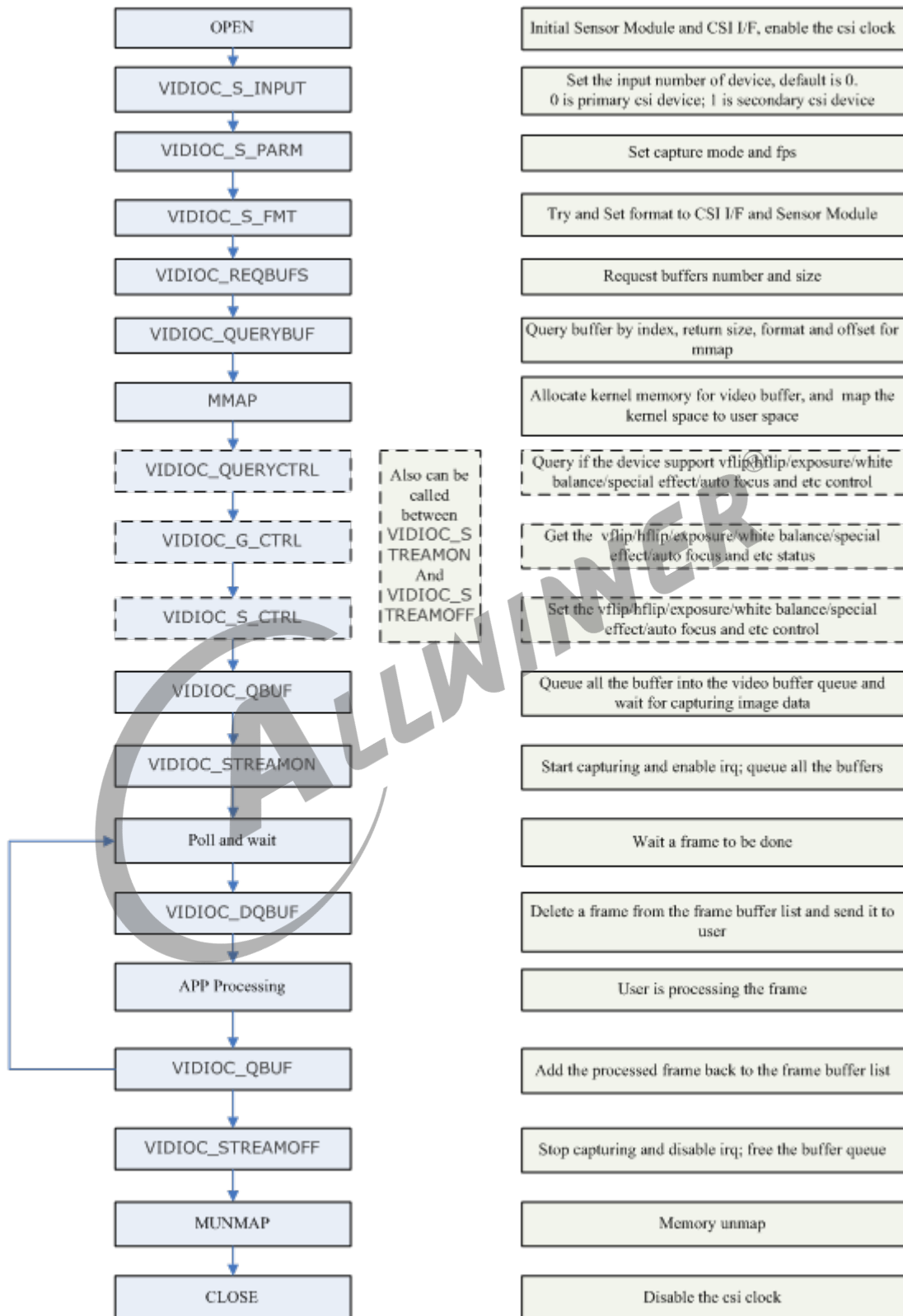
图 4-1: CSI 调用流程
