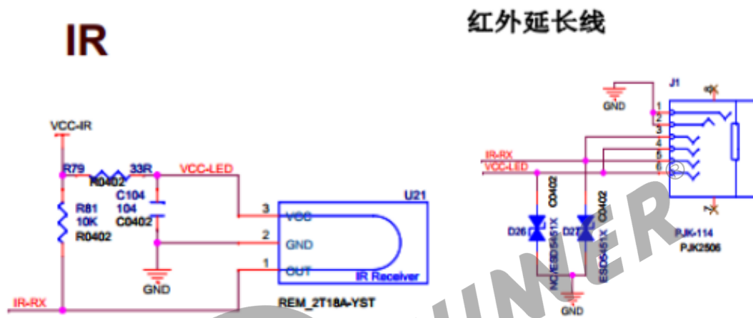
图 2-1: IR-RX 模块
