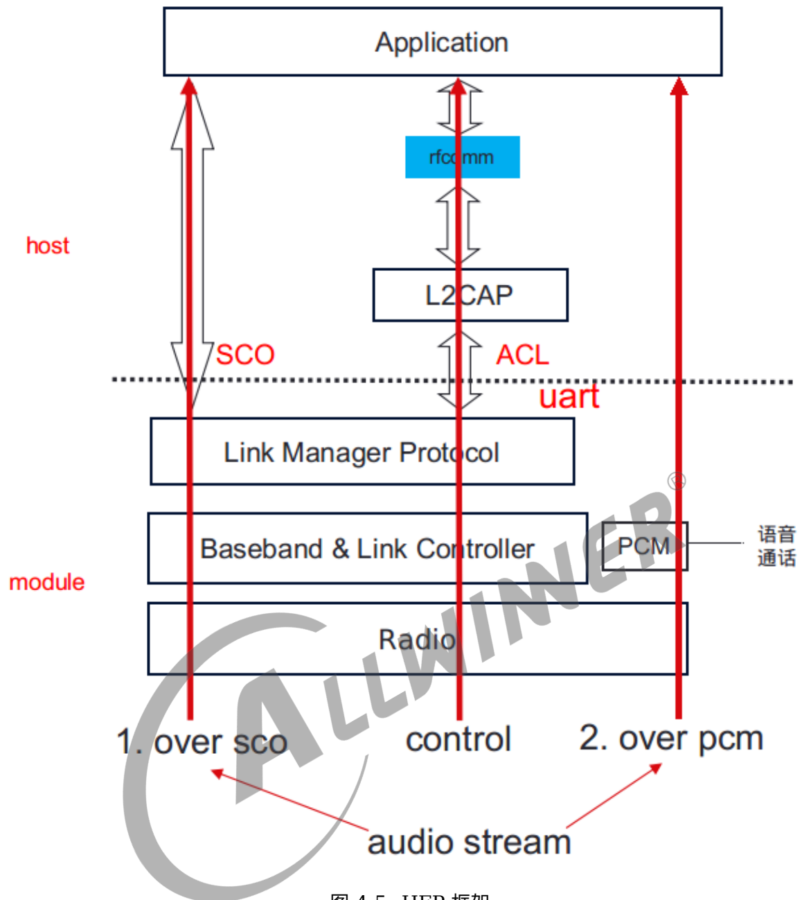
图 4-5: HFP 框架
