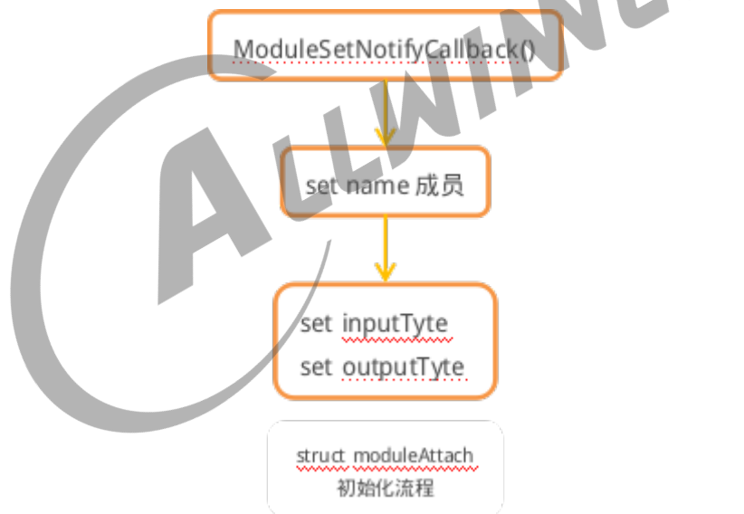
图 6-1: module init
