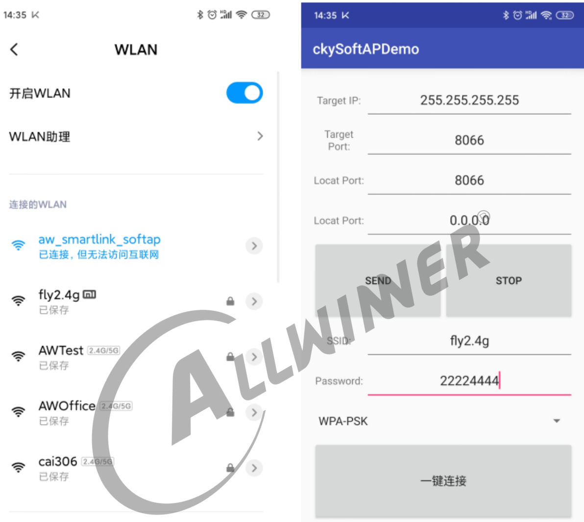
图 3-3: softap 配网
