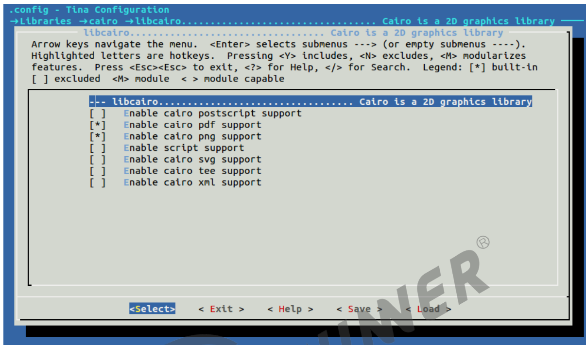
图 8-4: Cairo 选项
