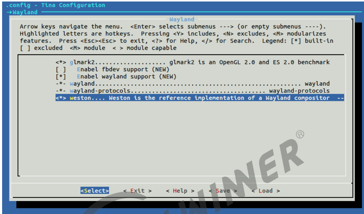
图 8-1: Wayland 选项
