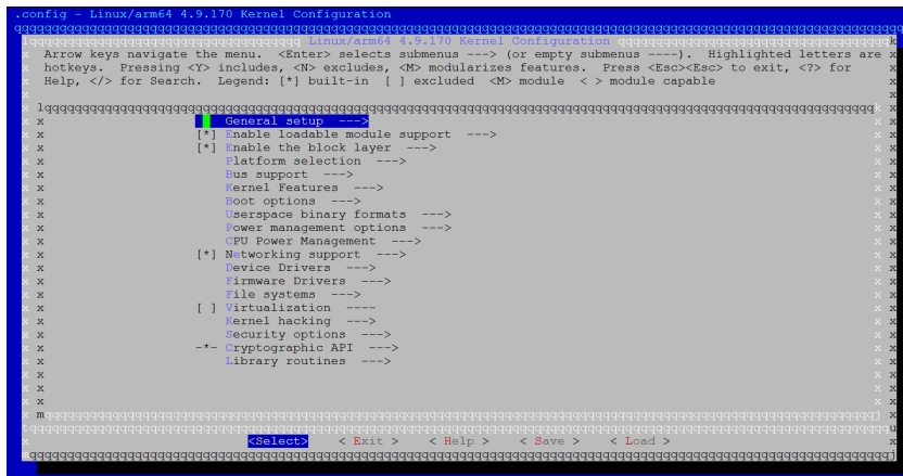
图 2-5: menuconfig 配置
