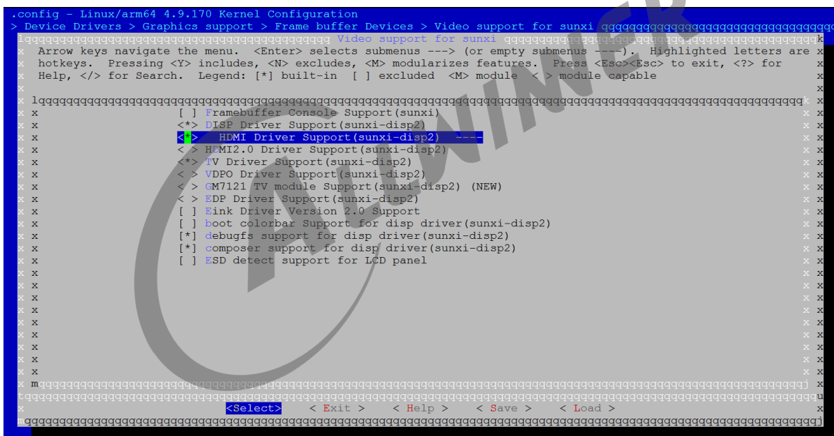
图 2-6: disp2 配置
